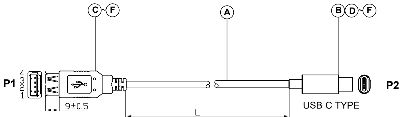
P1 USB A-TYPE(F)
