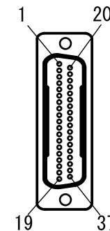
嵌合面から見た回路番号
