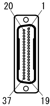
嵌合面から見た回路番号
