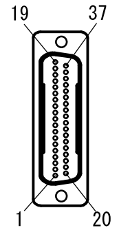
嵌合面から見た回路番号
