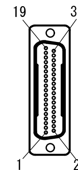
嵌合面から見た回路番号
