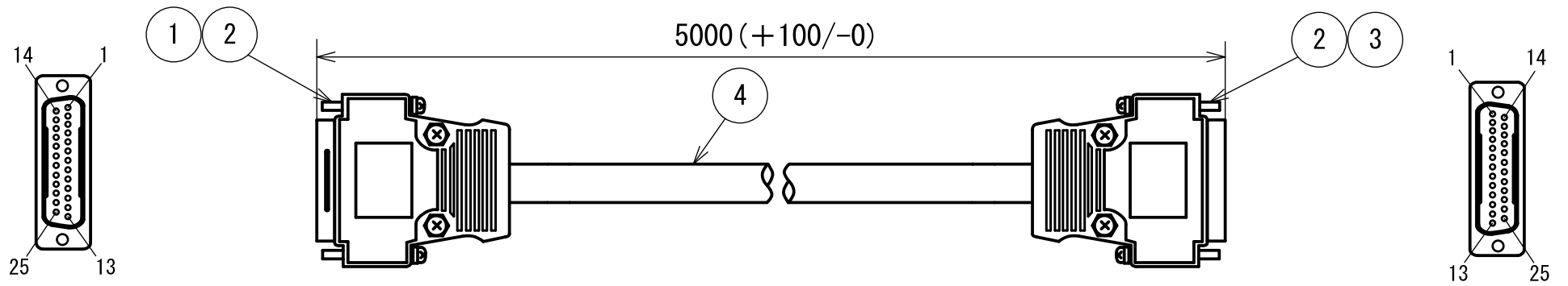
嵌合面から見た回路番号
