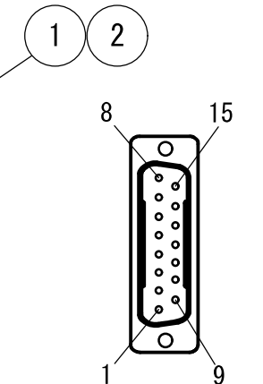
嵌合面から見た回路番号
